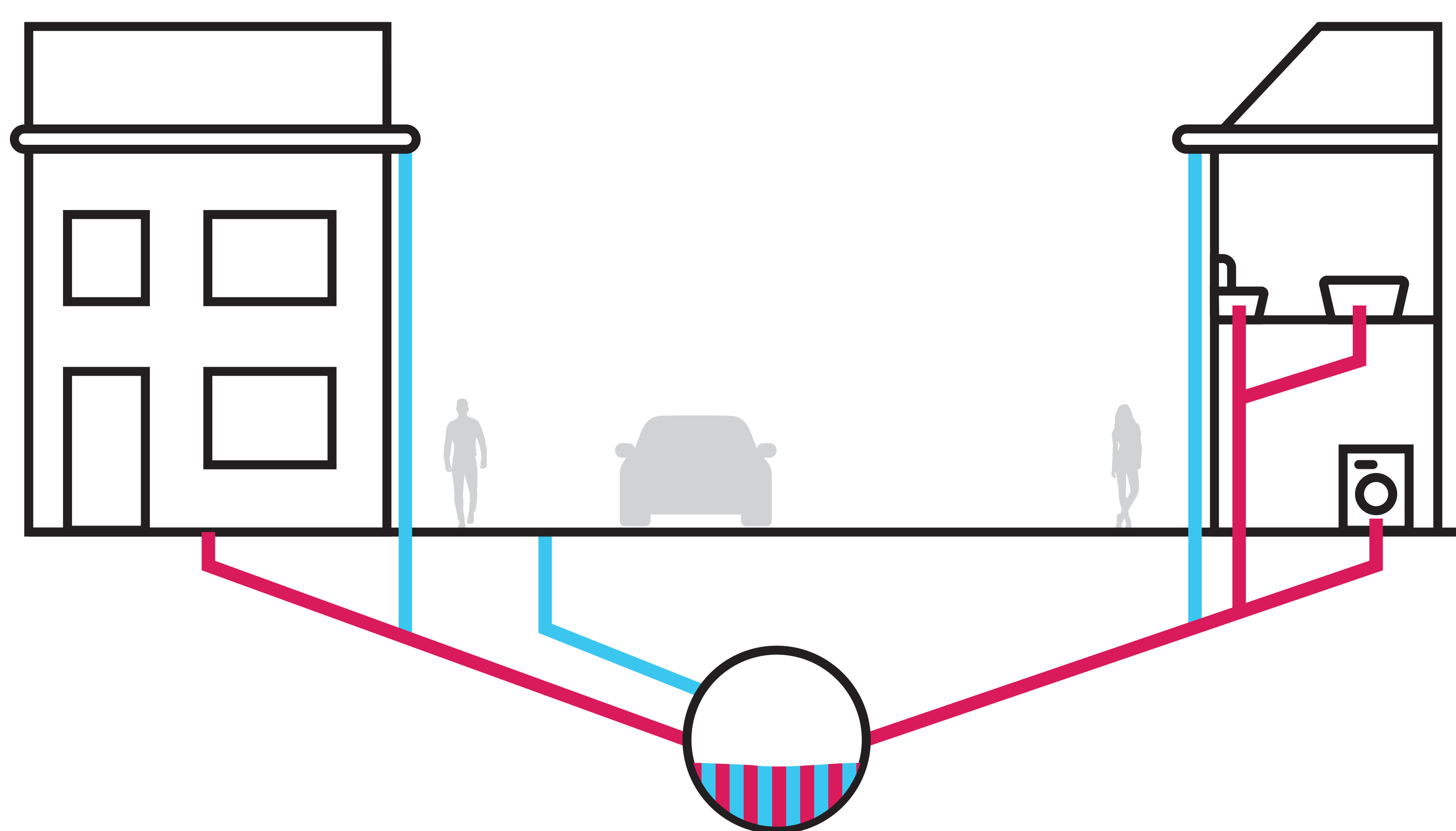
GEMENGD RIOLERINGSSTELSEL
